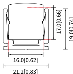
带金属弹片安装铝槽 型号: ASY-1617-A2(A4)NNXXX-MT
