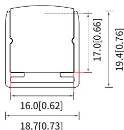
安装铝槽 型号: ASY-1617-A1(A3)NNXXX-MT
