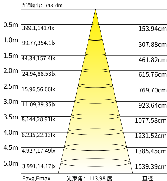
平均照度图
