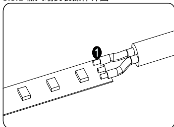
①. 将线与 PCB 板焊接起来;
