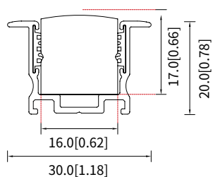
带硅胶条安装铝槽 (带翅) 型号: ASY-1617-A7NNXXX-MT
