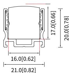
带硅胶条安装铝槽 型号: ASY-1617-A6NNXXX-MT
