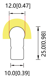
截面示意图:
