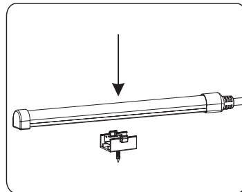
②. 将灯带慢慢压入安装铝槽;
