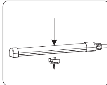
②. 将灯带慢慢压入安装卡;
