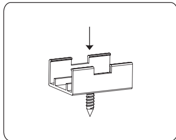
①. 将安装铝槽用螺丝固定在安装位置上;
