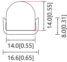
塑胶安装卡 型号: ASY-NDR1414-P1NNXXX-MT
