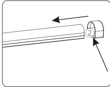
①. 堵头内部打上适量胶水, 再推入灯带;
