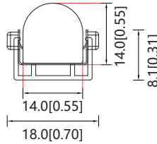
带金属弹片安装铝槽 型号: ASY-NDR1414-A2(A4)NNXXX-MT
