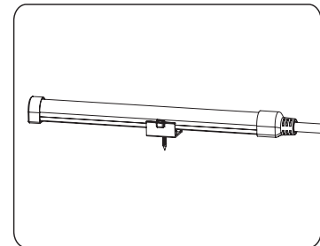
③. 灯带平整、牢牢低卡在安装铝槽上, 即可;
