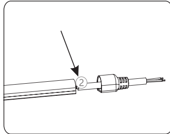
②. 先在堵头内部防胶水, 再推入灯带;
