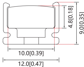
霓虹 + 型材后截面示意图:
