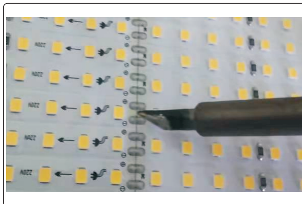
②.先用锡线润下烙铁头，迅速将烙铁头接近需要焊接的位置，切记烙铁头与PCB最长接触时间不超过3s。
