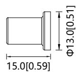
有孔堵头:
