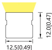
截面示意图:
