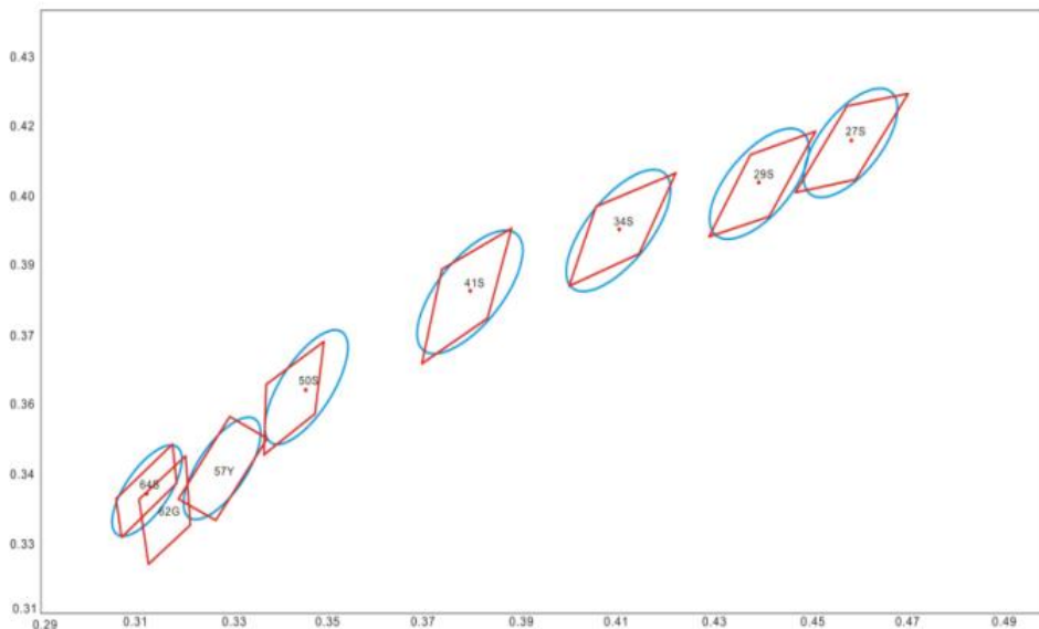
●分光打靶图 Chromaticity coordinates bin chart:
