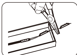
④ 剪切模组到所需的数量，并把剪切后的线头做好防水和绝缘处理。 △ 注意：剪切模组间的导线时，请居中剪切
